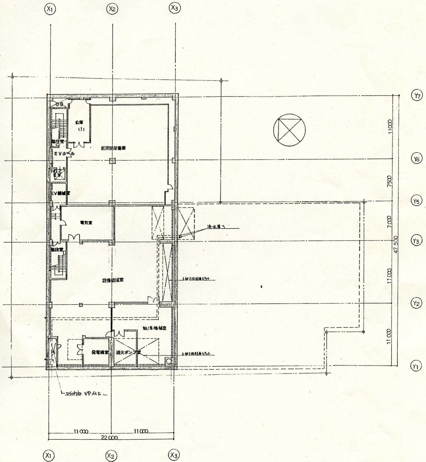
B2 階平面図
