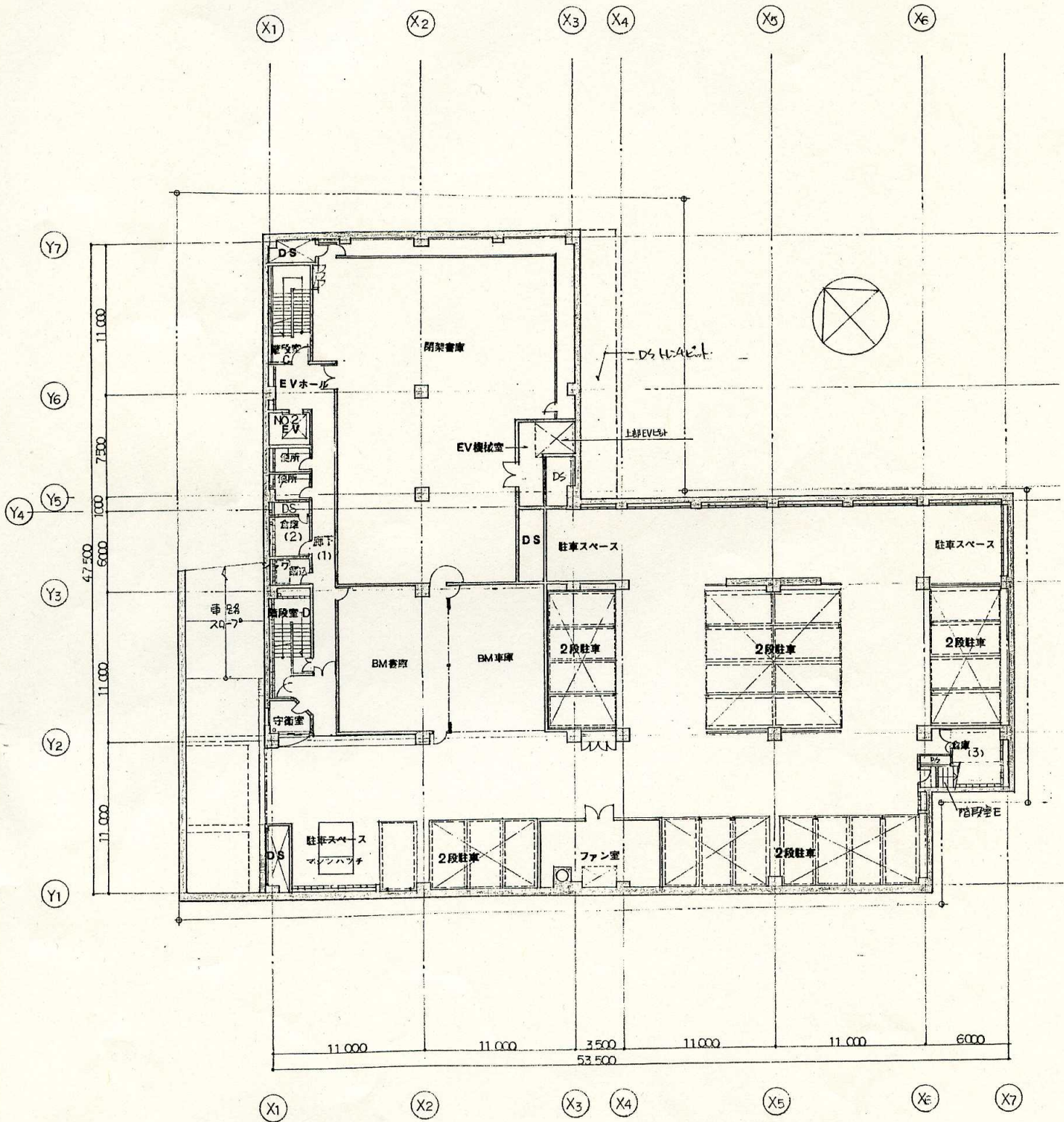
B1階平面図
