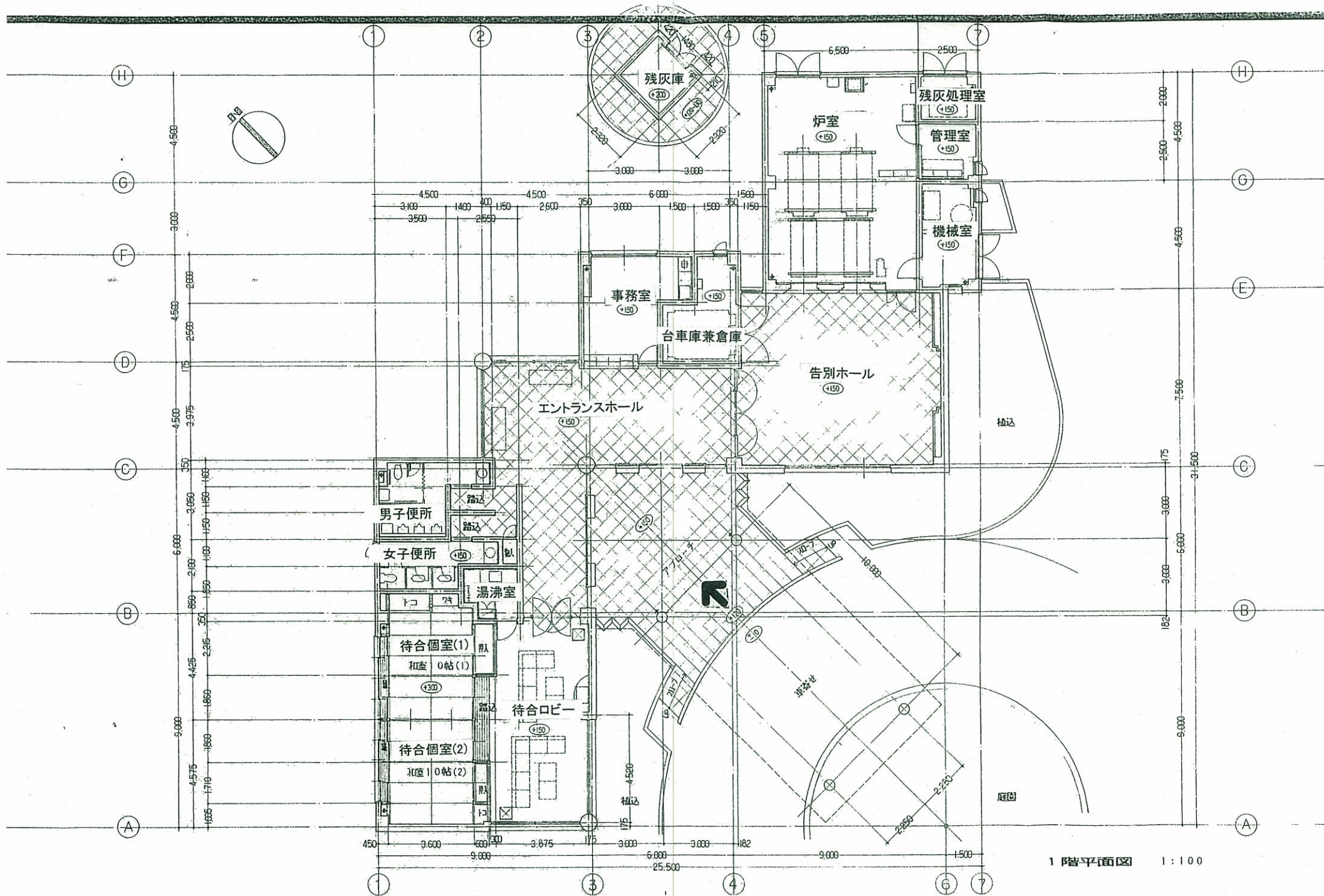
ふじさき苑 1階平面図
