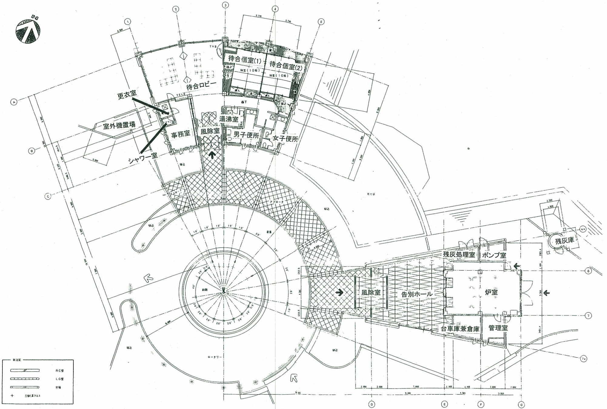
伯方斎場 平面図
