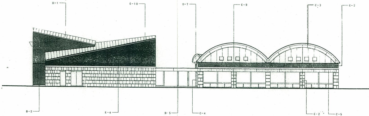
北側立面图
