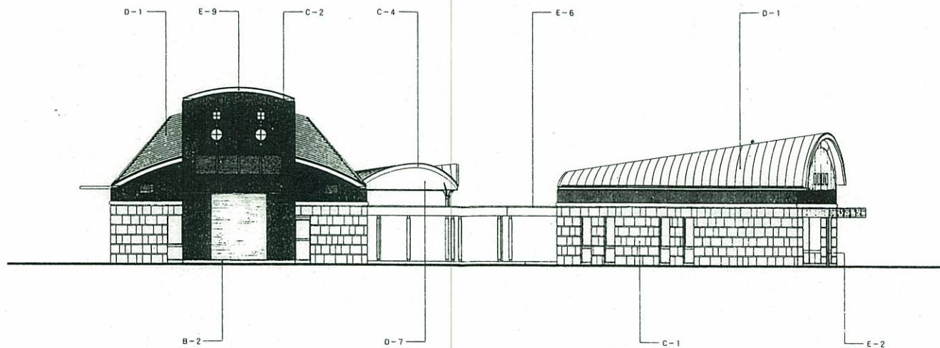
東側立面图
