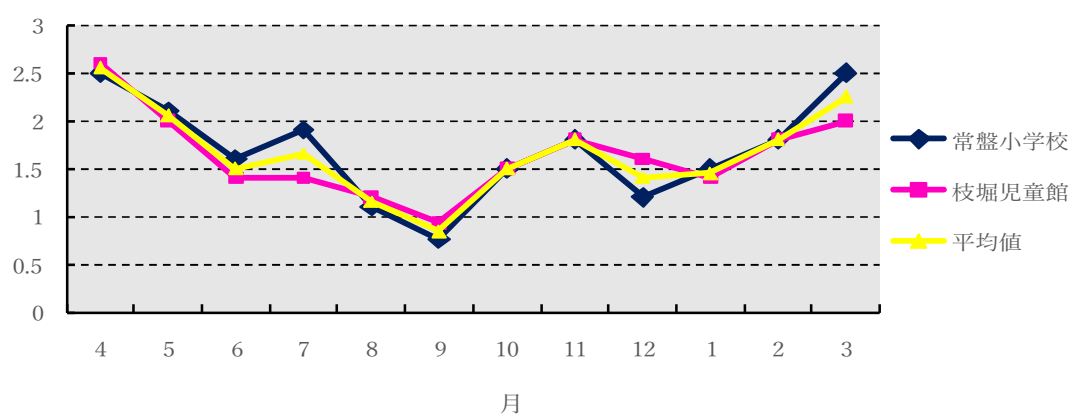
降下ばいじん 月別測定値 (単位：t/km 2 /月)
