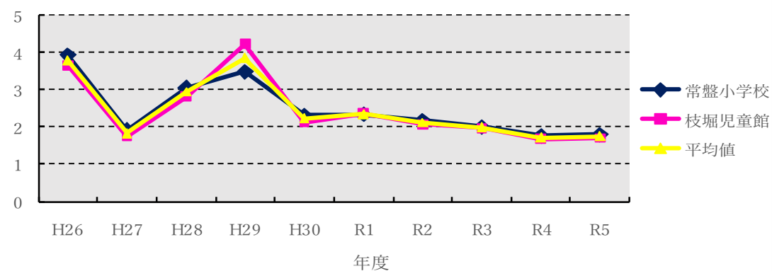
降下ばいじん 経年変化 (単位：t/km 2 /月)
