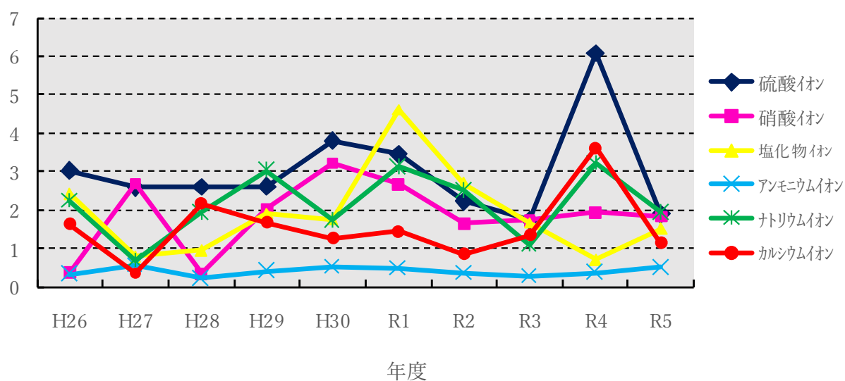
各種イオン 経年変化（単位： \mu\text{g/ml} ）
