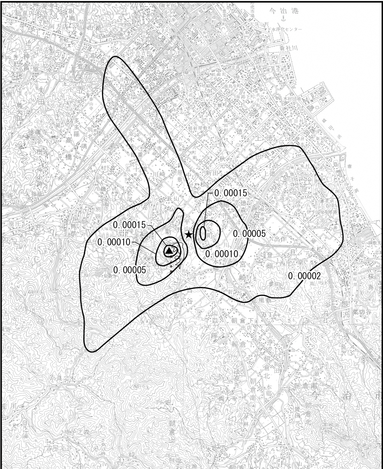
図 5.1.2-15(1) 大気汚染物質付加濃度予測結果 (ダイオキシン類、排ガス量最小時)
