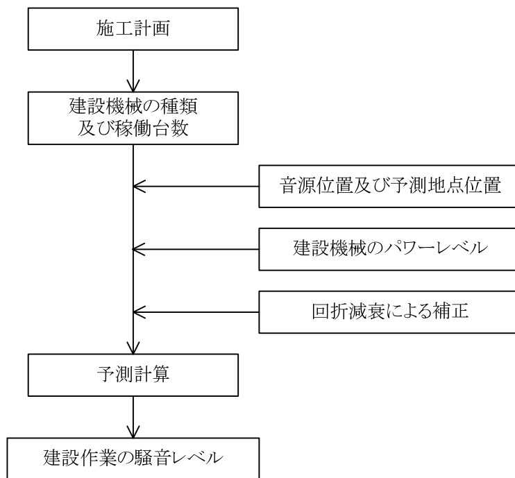
図 3.2.3-1 建設機械の稼働に伴う騒音の予測手順
