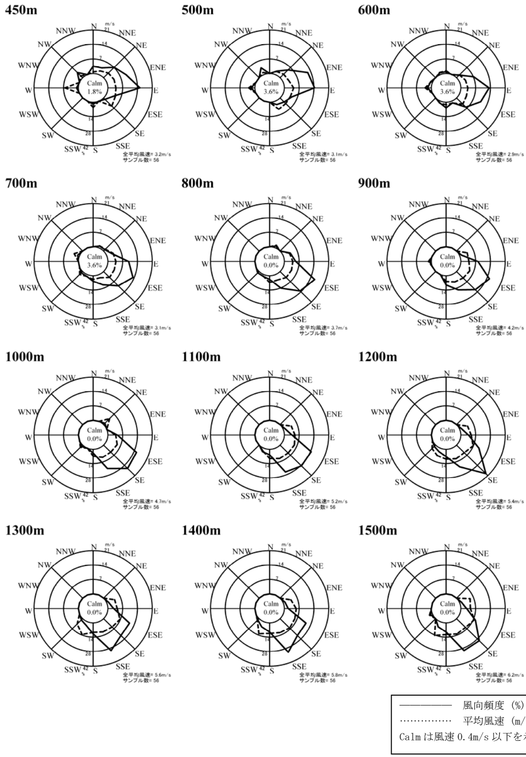
図 3.7.1-4(2) 高度別風配図(夏季)
