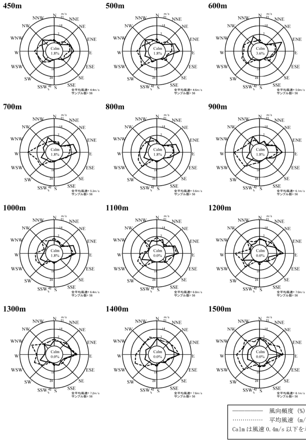
図 3.7.1-3(2) 高度別風配図(春季)
