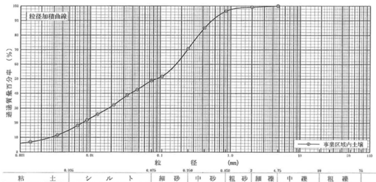
図 5.5.1-2 対象事業実施区域内の土壌の粒度組成
