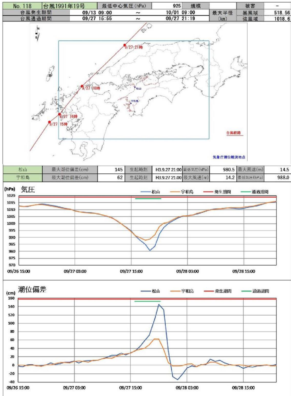
図4－1 平成3年台風19号の概要
