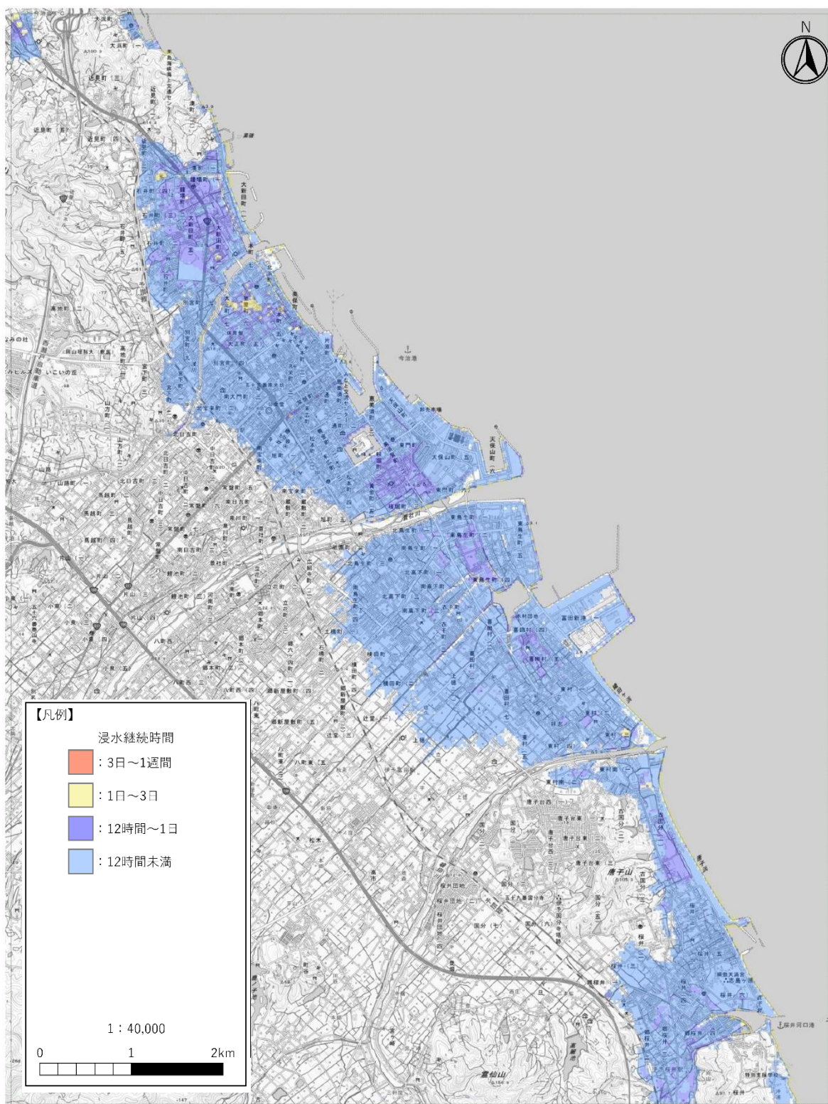
図4-4 愛媛県高潮浸水想定区域図 今治市 浸水継続時間
