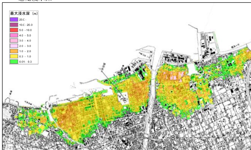
図 4-2 想定浸水深（南海トラフ巨大地震）
