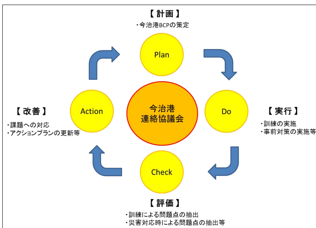
図 6-1 PDCAの概要
