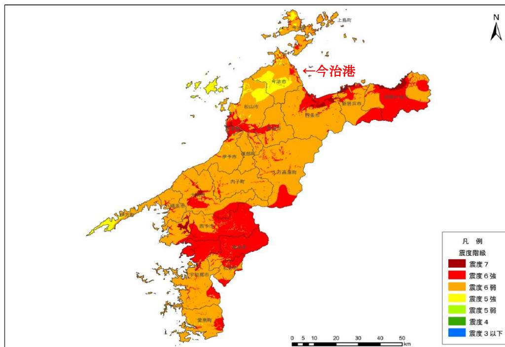
図 4-1 震度分布（南海トラフ巨大地震）
