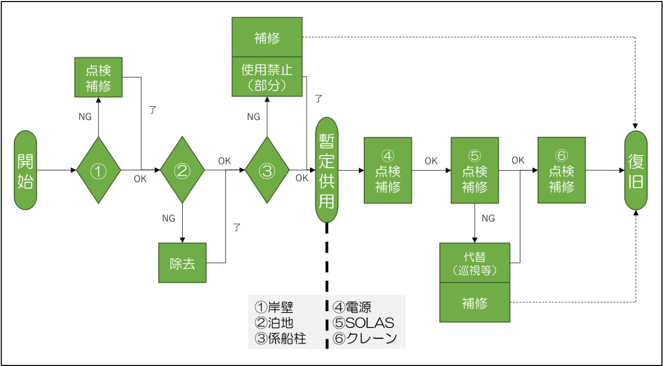
図 5-2 点検作業フローチャート
