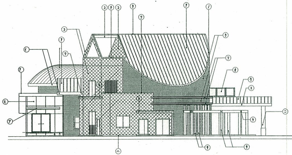
北立面図(改修後) 1/200
