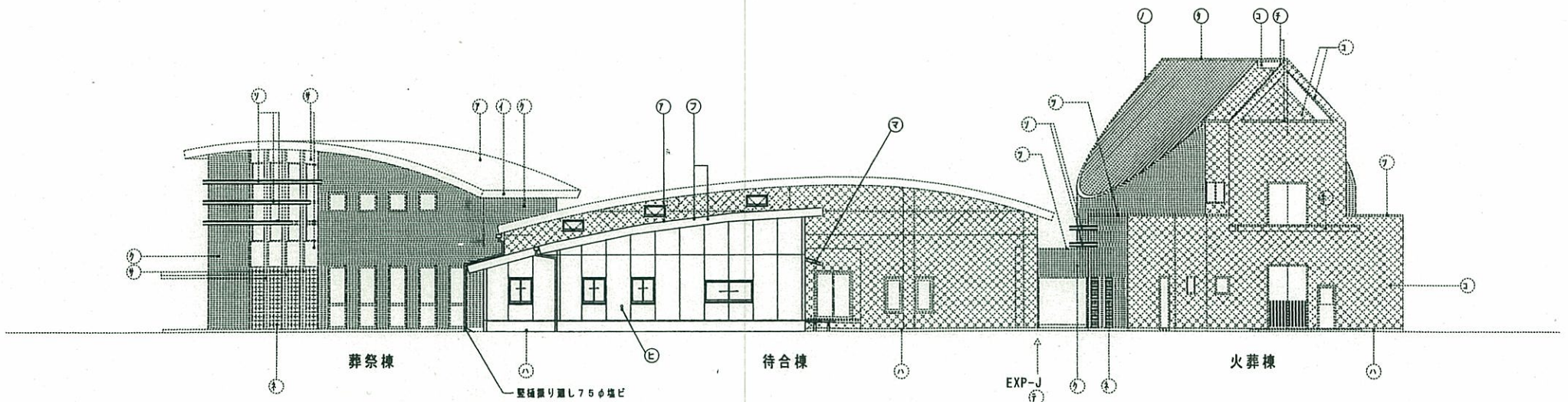
東立面図(改修後) 1/200
