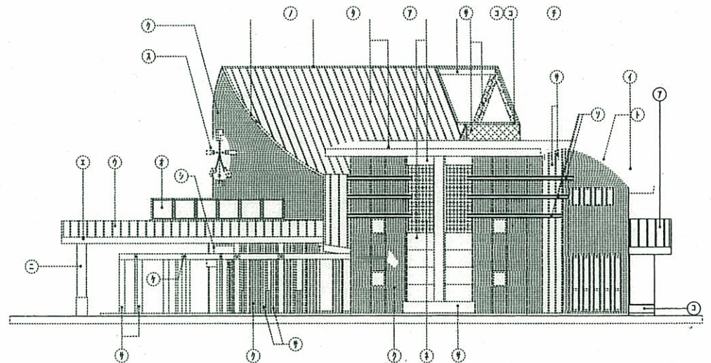
南立面図(改修後) 1/200
