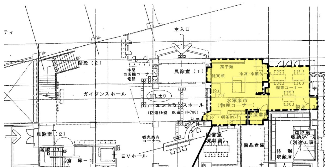
今治市村上水軍博物館物産コーナー（喫茶コーナーを含む）平面図
