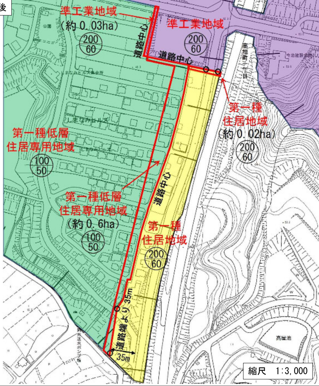
計画図 8
