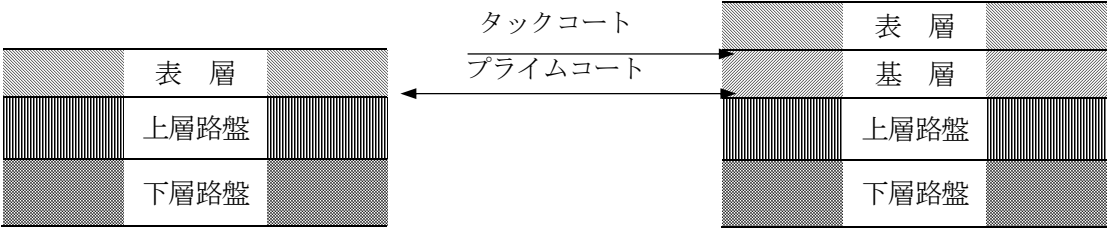
図－9 舗装標準断面図
