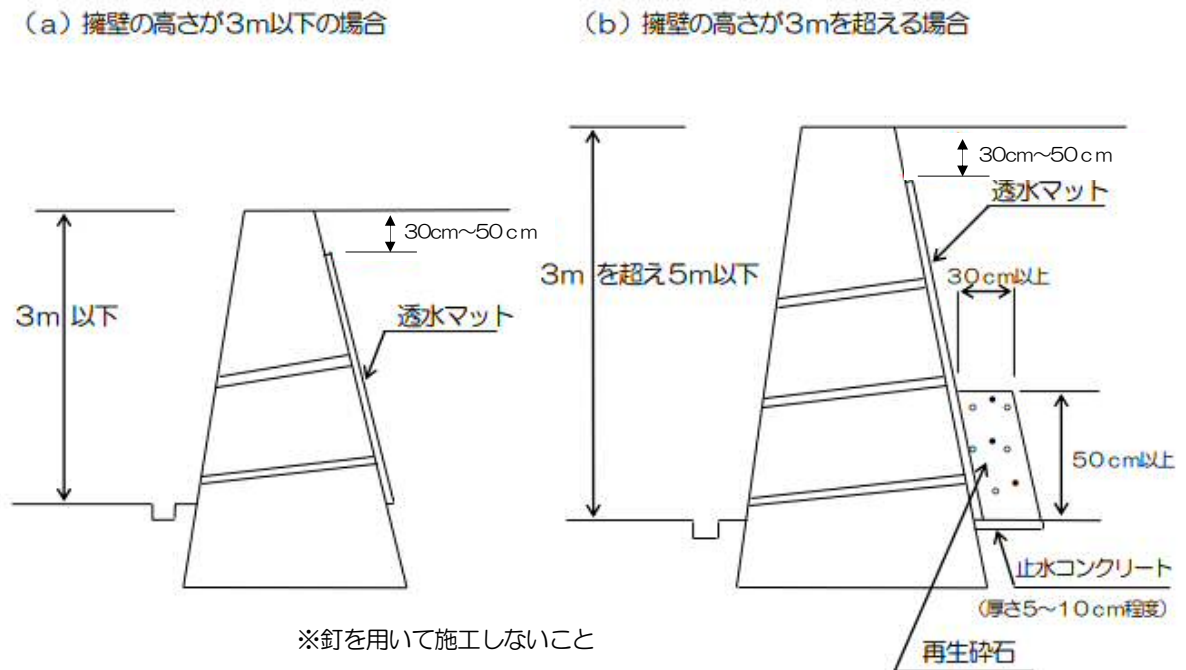
図－２６ 透水マットの取付断面図
