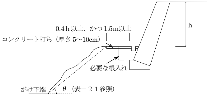
図－２３ がけ上に設置する擁壁の位置
