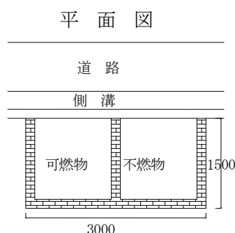
ごみ集積施設 標準構造図 (参考)
